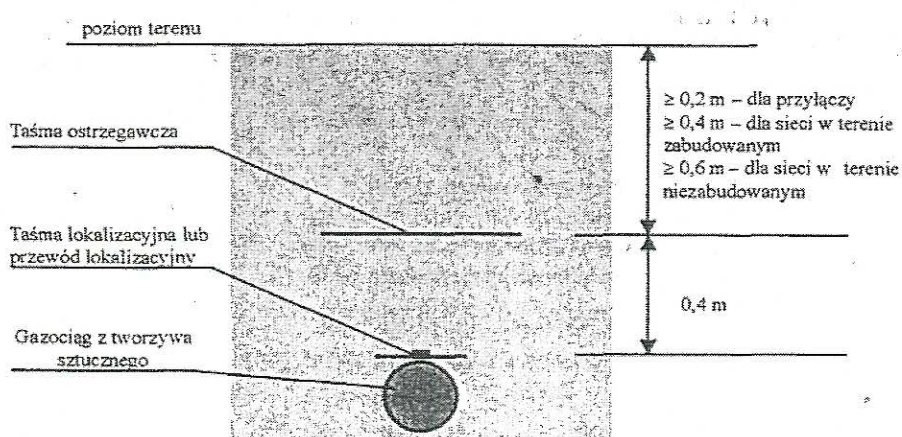
Rys. nr 8. Sposoby oznakowania gazociągów z tworzyw sztucznych
